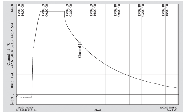
Wykres rzeczywisty procesu odprężania płyt Original stress relieving process example
